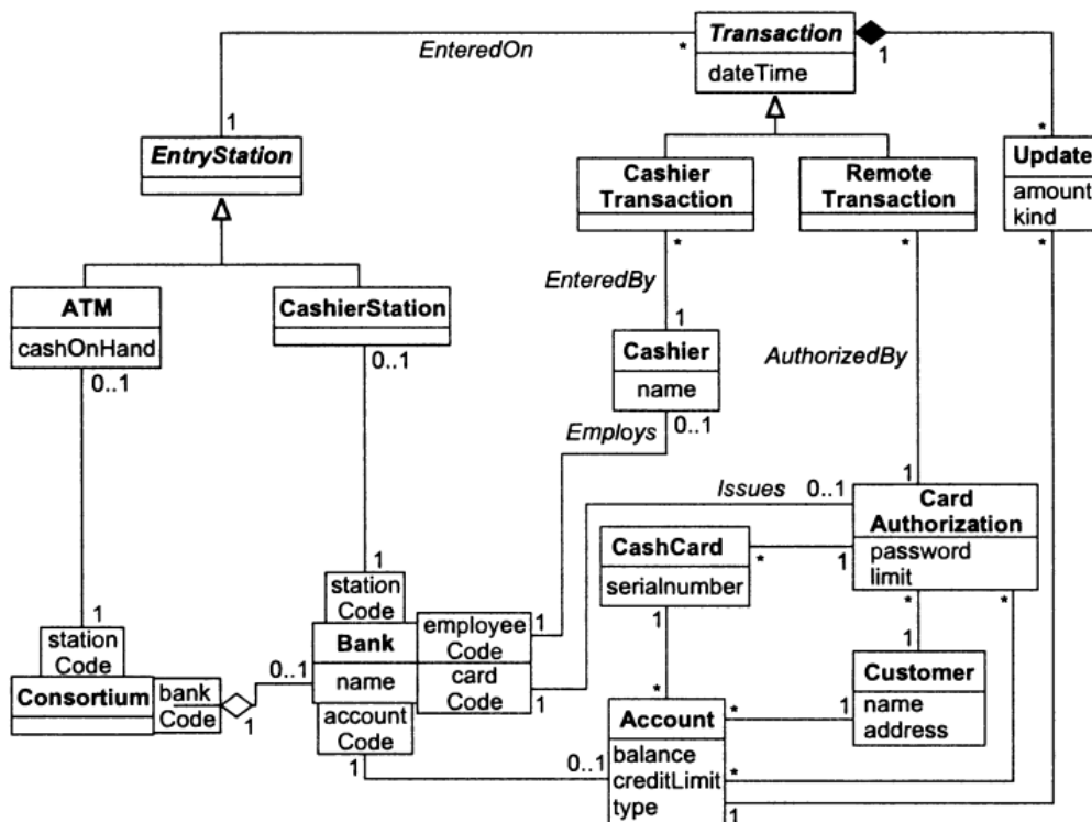
Рис. 4.6 – Модель классов банкоматов после очередных исправлений
