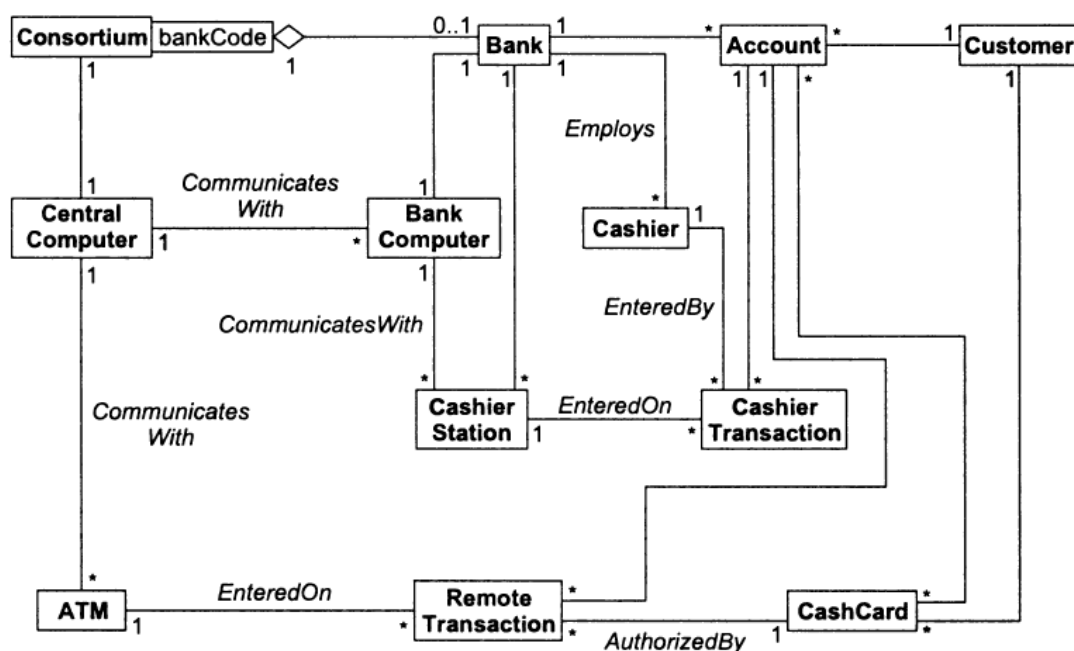
Рис. 4.3 – Исходная диаграмма классов для банкомата
