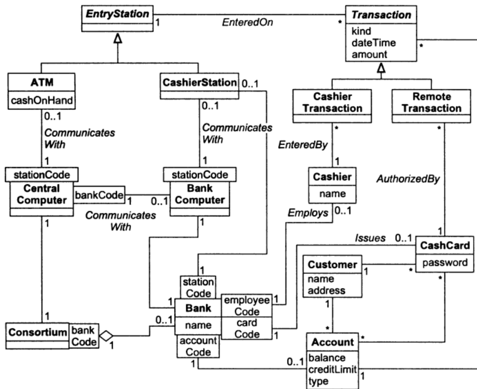
Рис. 4.5 – Преобразованная модель классов банкомата
