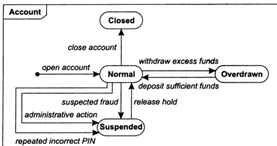
Рис. 4.7 – Модель состояния предметной области
