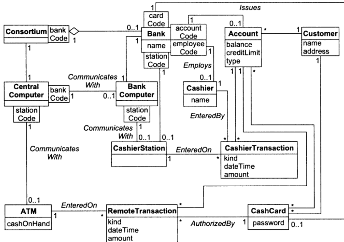
Рис. 4.4 – Модель классов банкомата с атрибутами
